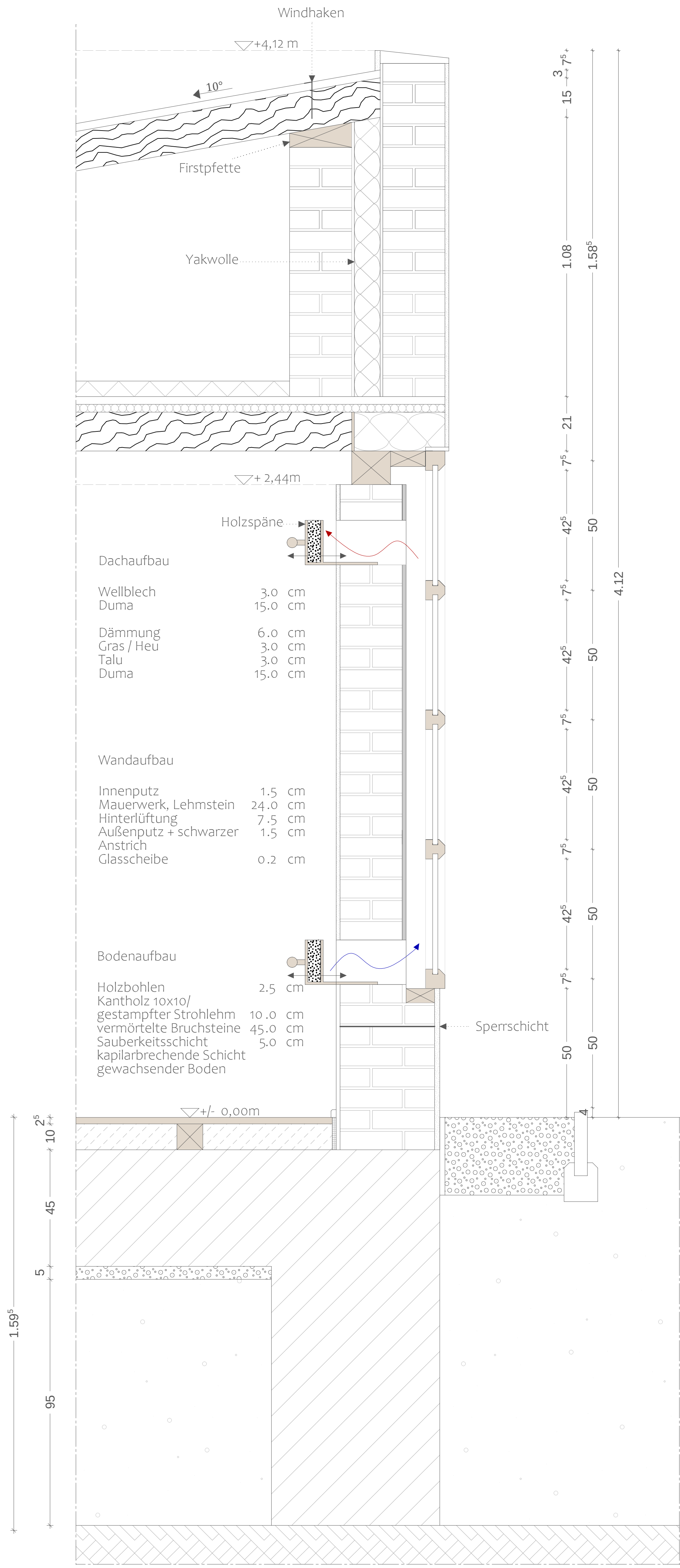
| DETAIL B. Fensteranschluss 1:10
