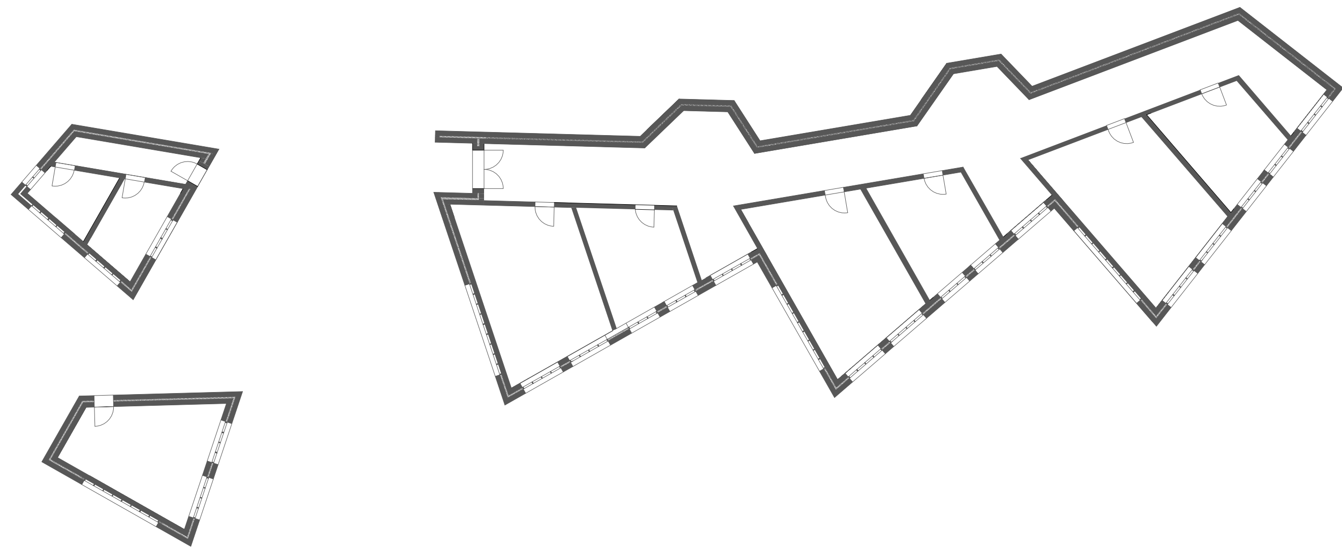
| Gesamt Grundriss 1:200
