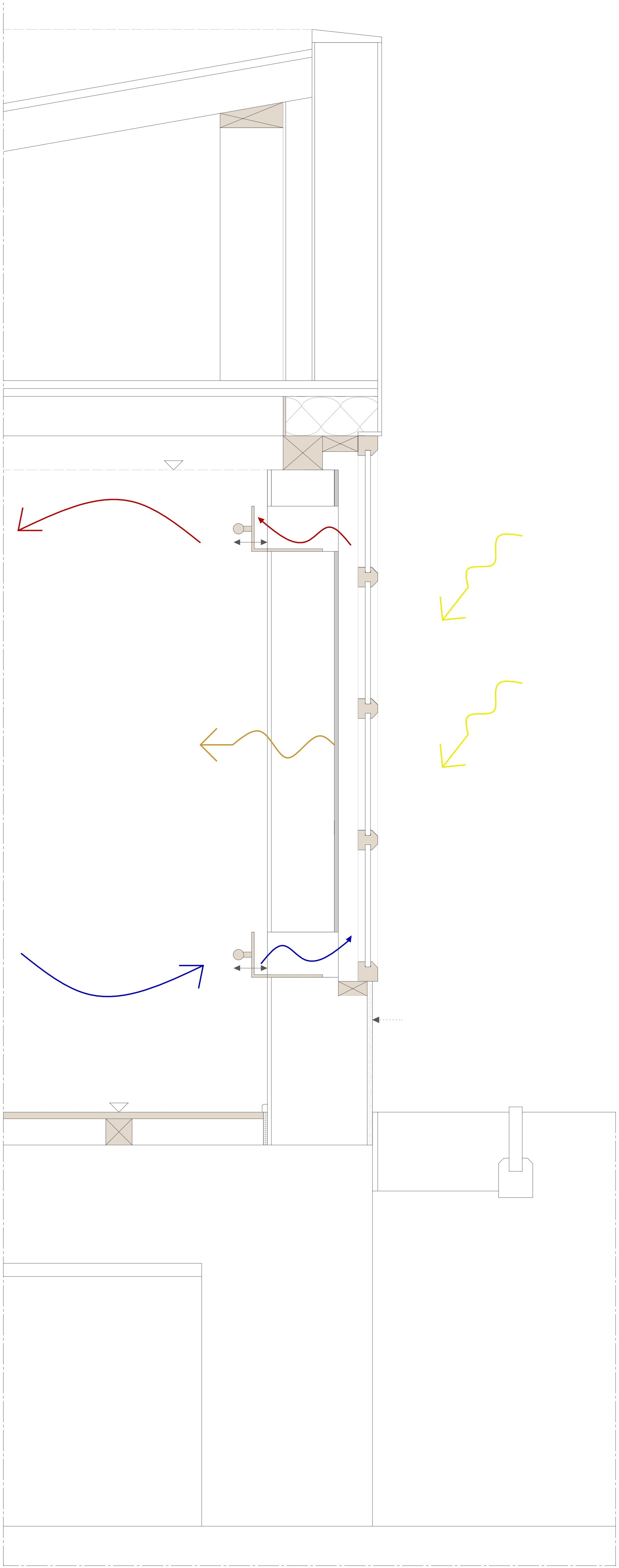
KONVEKTION LUFTAUSTAUSCH DURCH TROMBEWAND
