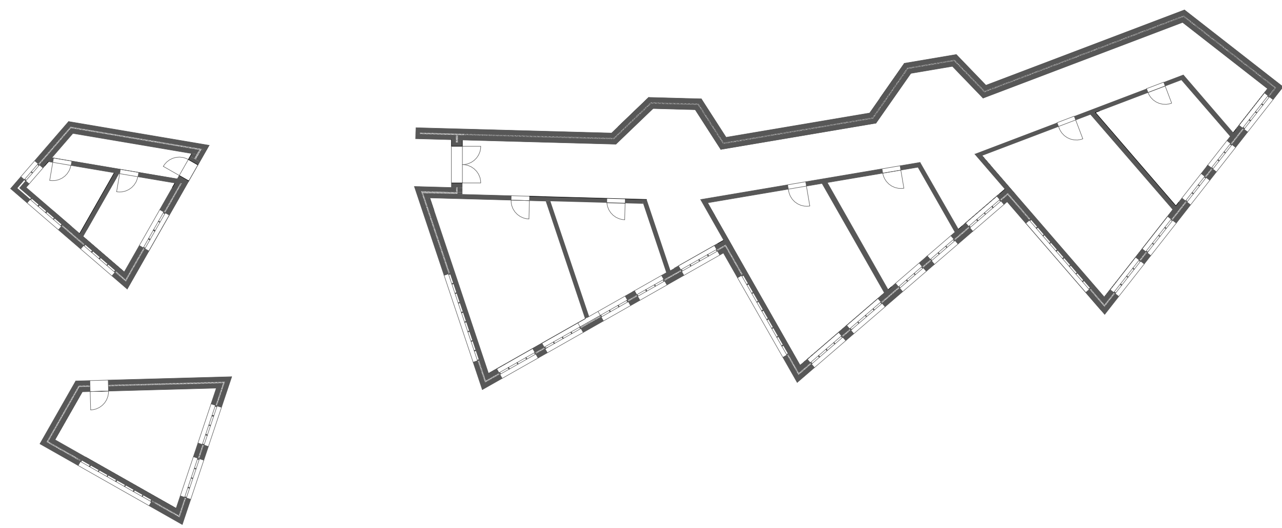
| Gesamt Grundriss 1:200
